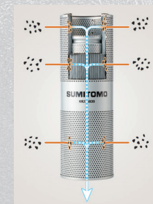
リターンフィルタの詳細
